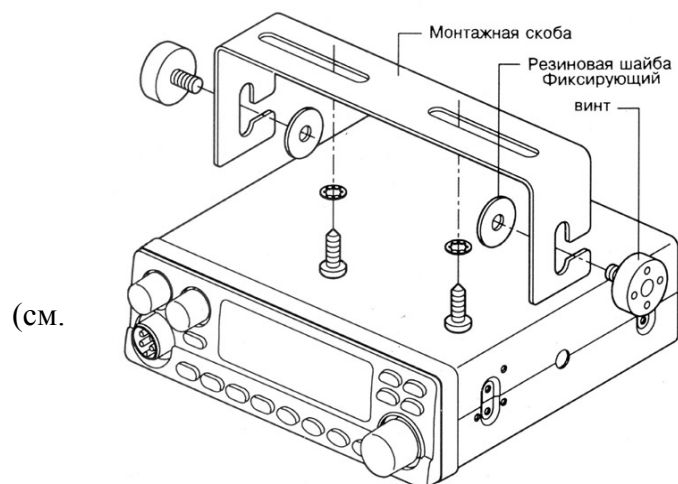
Рис.1. Крепление радиостанции при помощи монтажной скобы.
